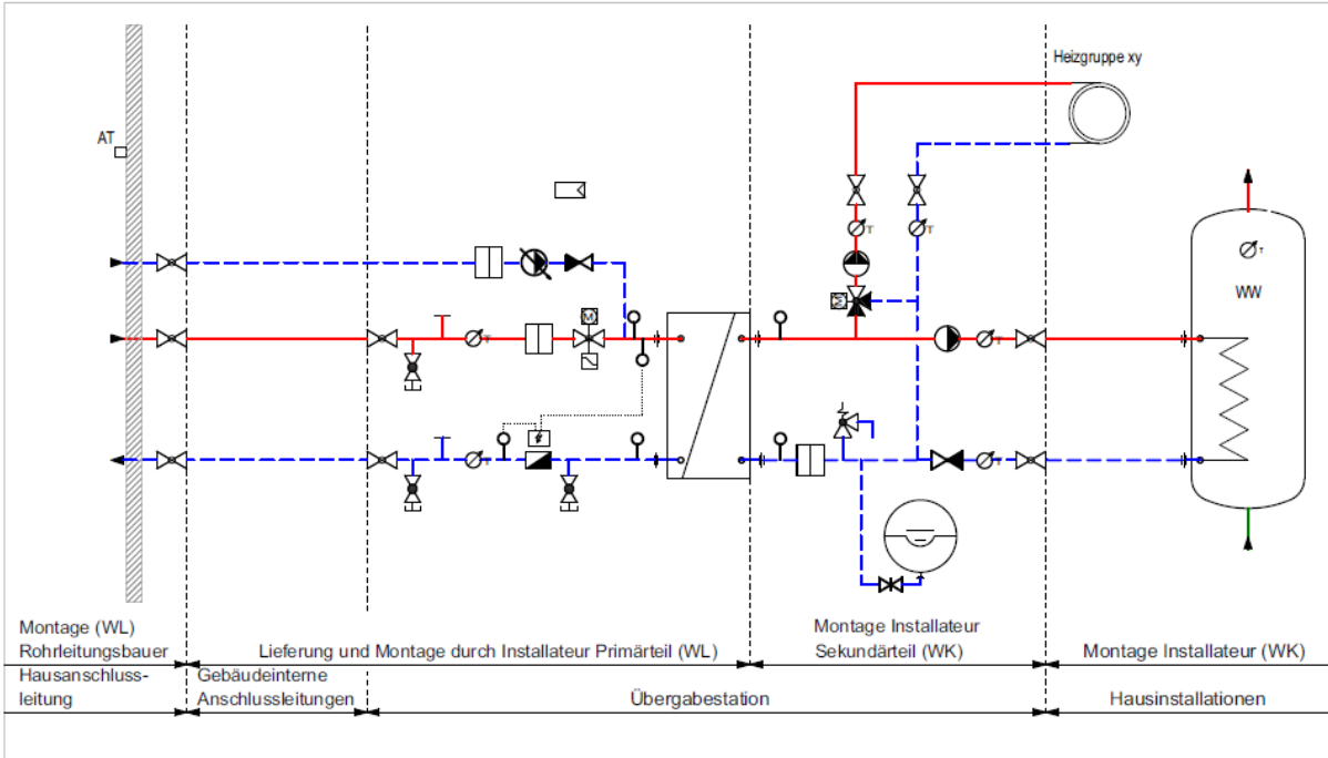
Abbildung 8 Muster-Prinzip-/Hydraulikschema Dreileiter-Station
