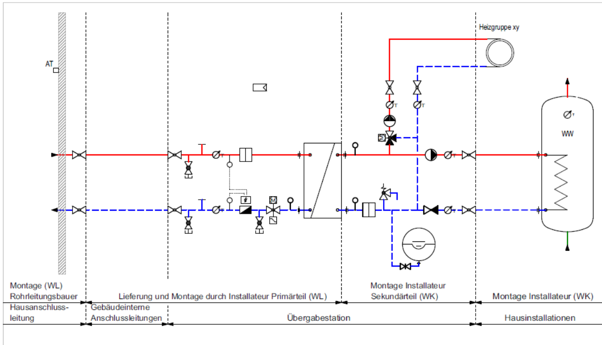
Abbildung 4 Muster-Prinzip-/Hydraulikschemata Variante 1, Registerwasserewärmer
