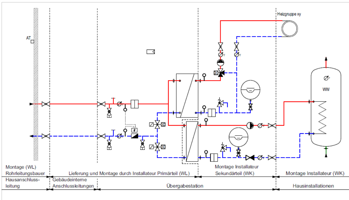
Abbildung 7 Muster-Prinzip-/Hydraulikschemata Variante 4, Magroladung mit direkter Fernwärmeeinbindung
